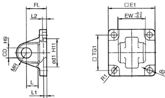
Fijación osc. macho trasera C
