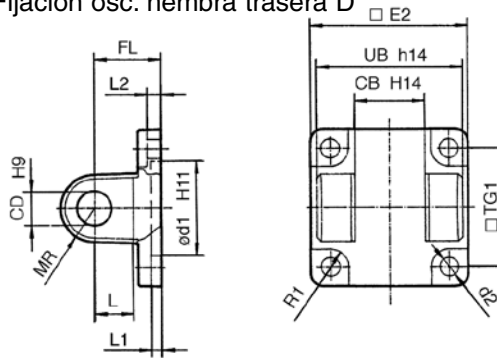
Fijación osc. hembra trasera D
