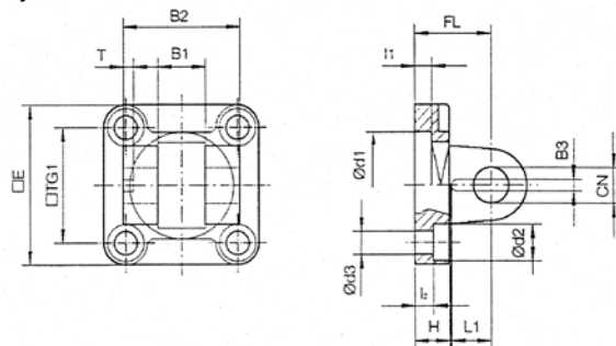
Fijación osc. macho trasera CS
